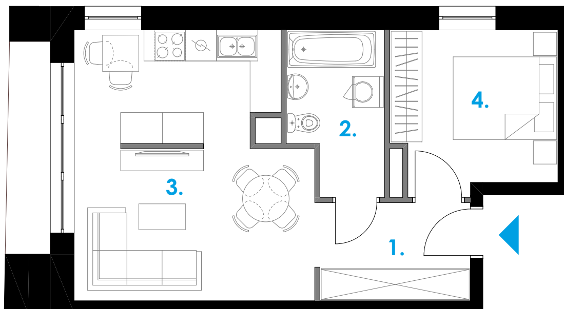
RZUT MIESZKANIA SKALA: 1:75
